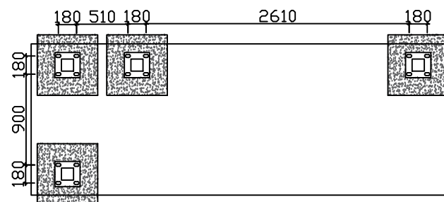
正视图
