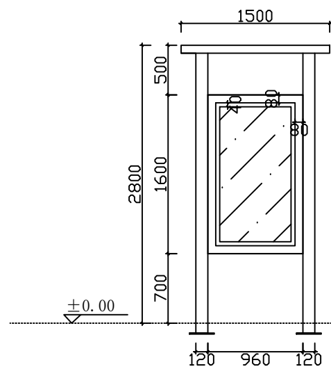
左视图
