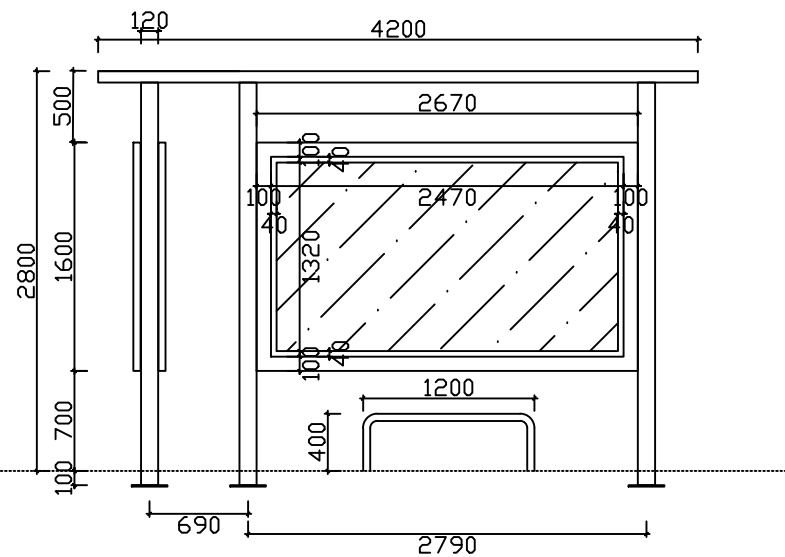
正视图
